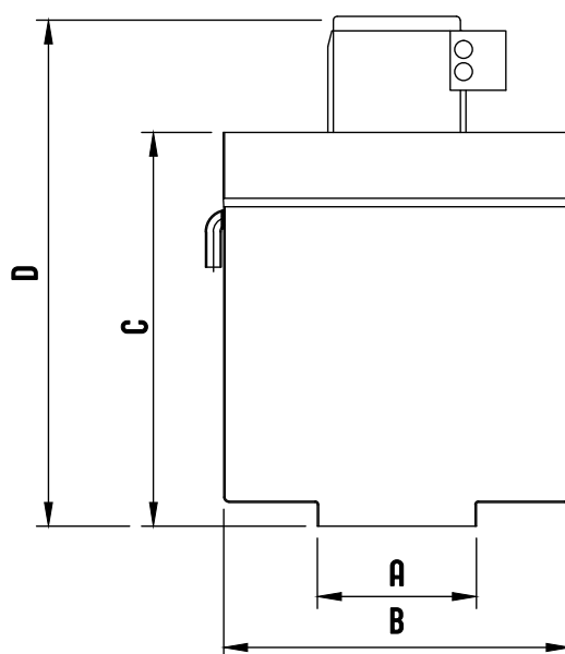
DIMENSÕES : EXAUSTORES EN - VERTICAIS E HORIZONTAIS
